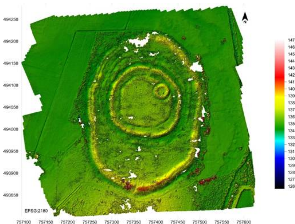
Ryc. 3. Dzięcioły, gm. Łosice. Grodzisko „Dawne Okopy”, rozplanowanie umocnień obronnych (oprac. M. Bogacki)
